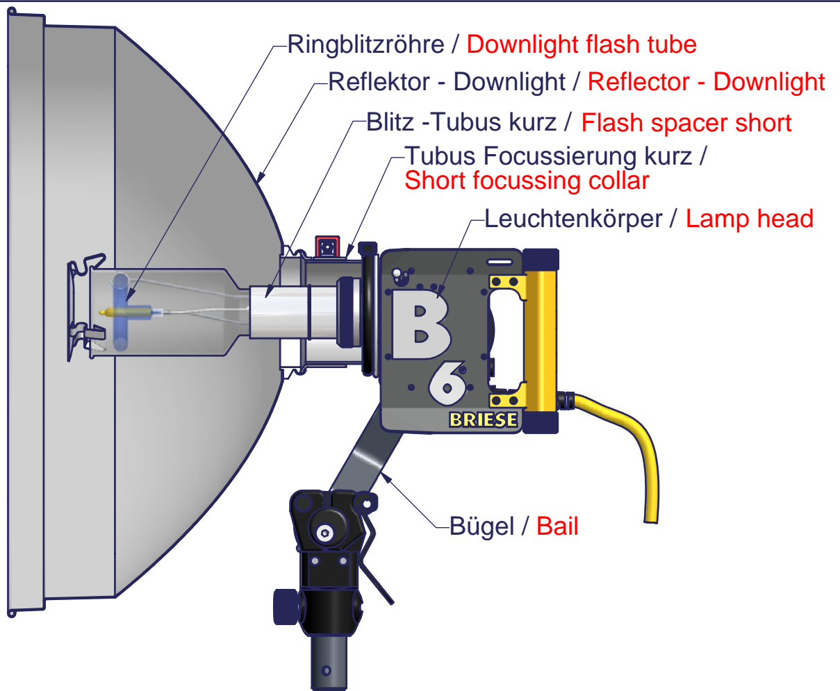
Aufbau der Downlightleuchte / set up Downlight reflector
